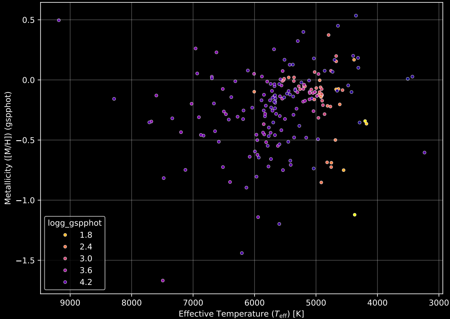
APOGEE DR17 Field: [074-35_MGA] Stellar Population Parameters (n= 202)
